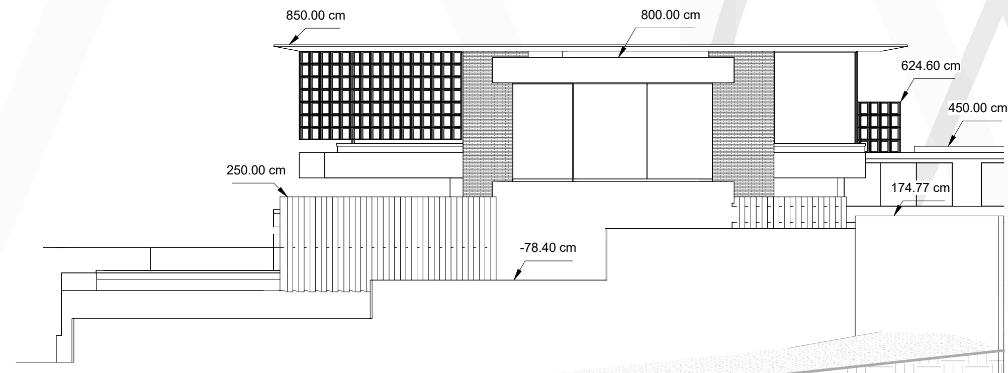
Elévation Ouest
