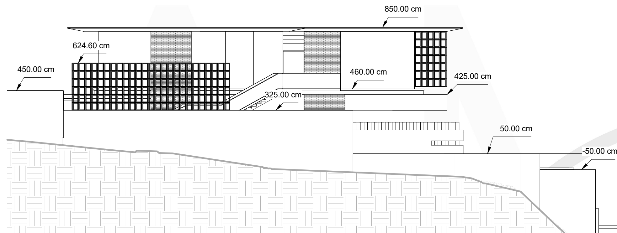
Elévation Est
